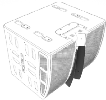
ANT-FLG60 Flanges de directivité à 60° pour M210
