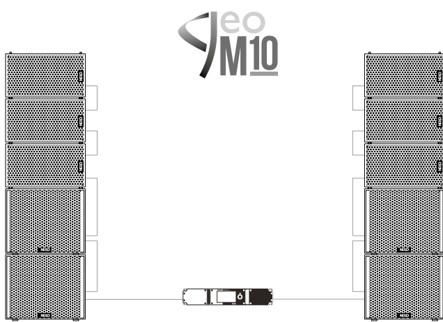
NXAMP4X2 MK2 alimentant 3 x GEO M10 et 2 x MSUB15 par côté
