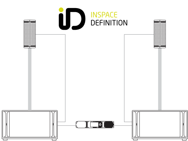
NXAMP4X1 MK2 alimentant 1 x ID24 et 1 x IDS110 Sub par côté
