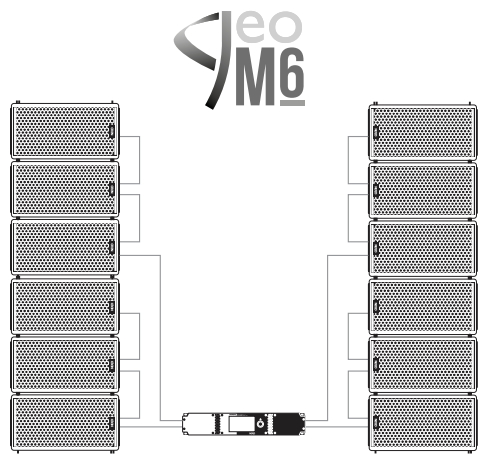
NXAMP4X1 MK2 alimentant 6 x GEO M6 par côté
