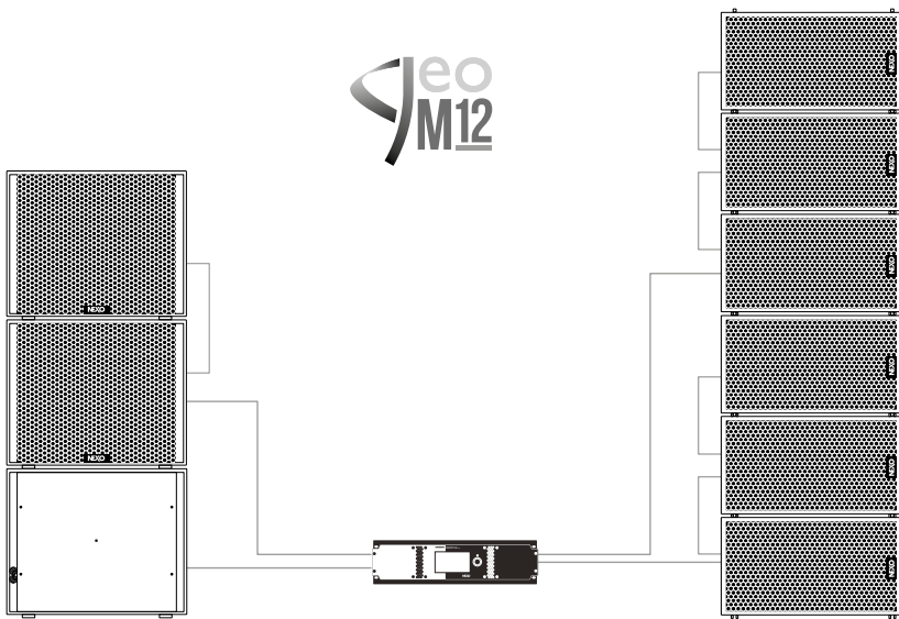
NXAMP4X4 mk2 alimentant 3 x MSUB18 (dont un en mode cardio) et 6 x GEO M12
