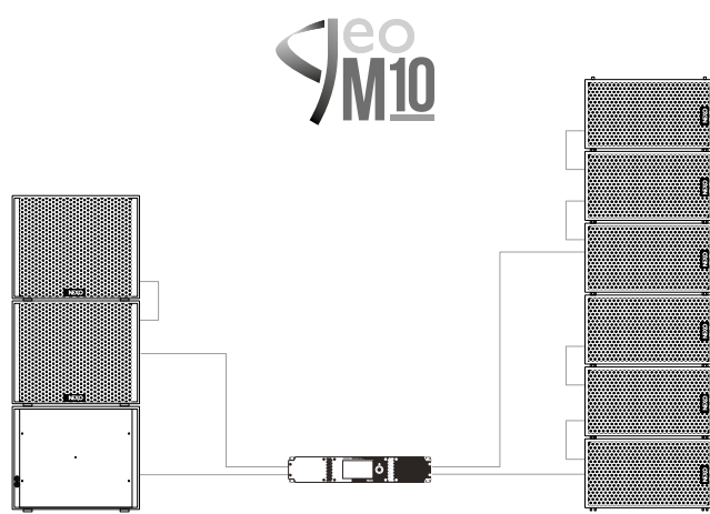
NXAMP4X2 MK2 alimentant 3 x MSUB15 (dont un en mode cardi-oïde) et 6 x GEO M10
