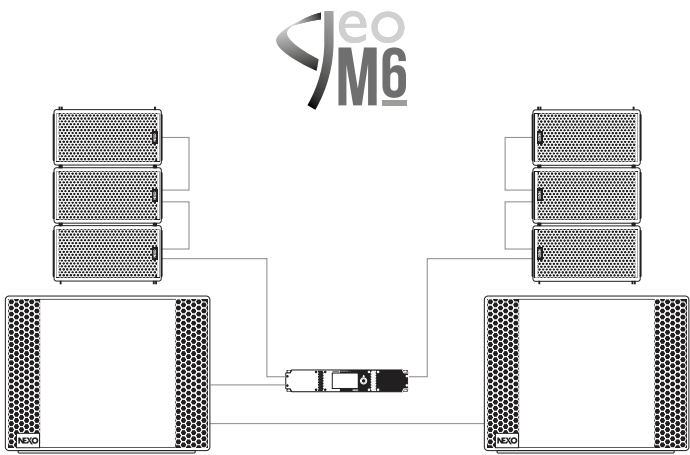
NXAMP4X1 MK2 alimentant 3 x GEO M6 par côté et 2 x LS18 en mode mono bridgé
