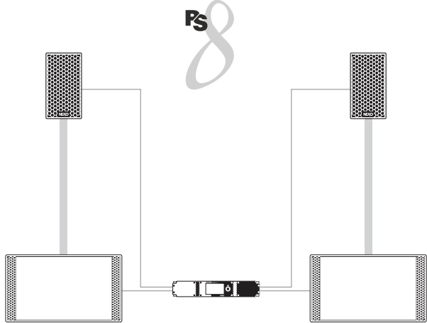
NXAMP4X1 MK2 alimentant 1 x PS8 et 1 x LS400 Sub par côté
