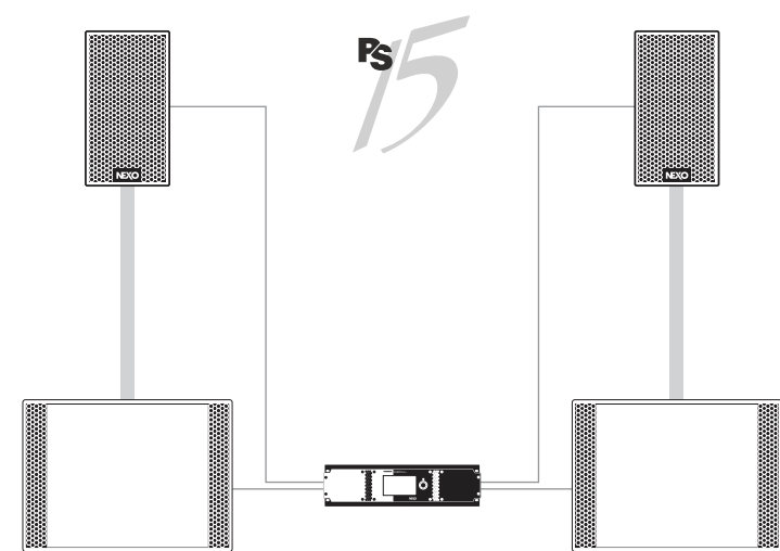
NXAMP4X4 mk2 alimentant 2 x PS15 et 2 x LS18 par côté
