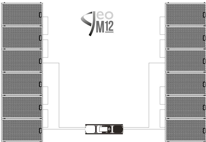
NXAMP4X4 mk2 alimentant 6 x GEO M12 par côté
