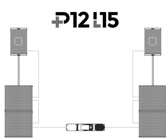
NXAMP4X2 MK2 alimentant 1 x P12 et 2 x L15 par côté
