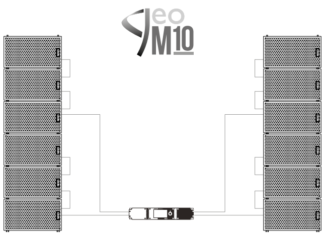
NXAMP4X2 MK2 alimentant 6 x GEO M10 par côté
