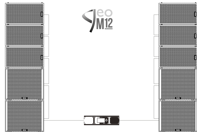
NXAMP4X4 mk2 3 x GEO M12 et 2 x MSUB18 par côté
